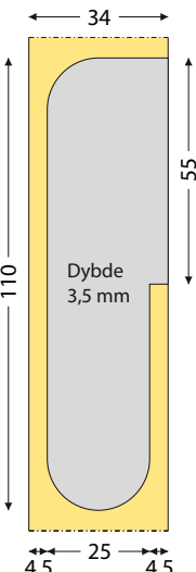
Type 12. Bladhængsel ASSA 3228.
