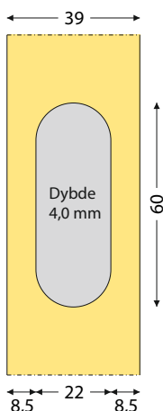
Type 03. Indstikshængsel metaldel.
