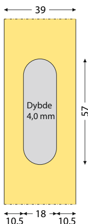
Type 04. Indstikshængsel metaldel.
