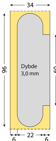
Type 09. Bladhængsel IPA 11251.
