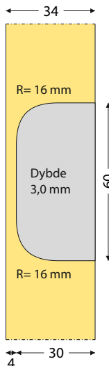
Type 10. Bladhængsel symetrisk.
