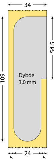
Type 11. Bladhængsel usymetrisk.
