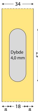
Type 07. Indstikshængsel metaldel.
