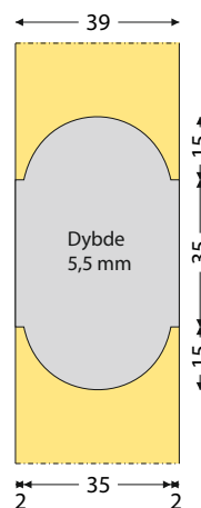
Type 13. Indstikshængsel plastdel.
