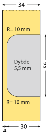
Type 05. Indstikshængsel plastdel.
