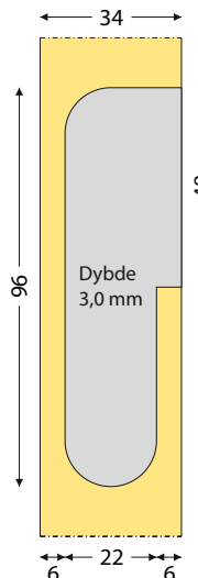
Type 14. Bladhængsel usymetrisk.
