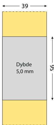
Type 02. Indstikshængsel plastdel.
