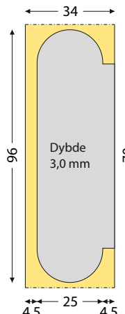
Type 08. Bladhængsel symetrisk.
