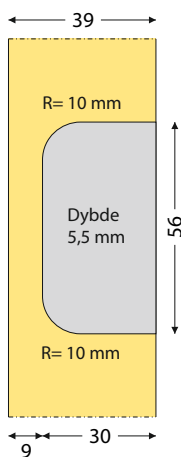
Type 01. Indstikshængsel plastdel.
