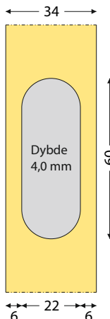
Type 06. Indstikshængsel metaldel.
